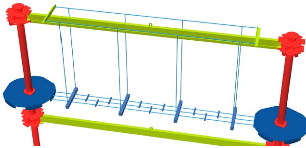
E120: Three Line Stirrups
